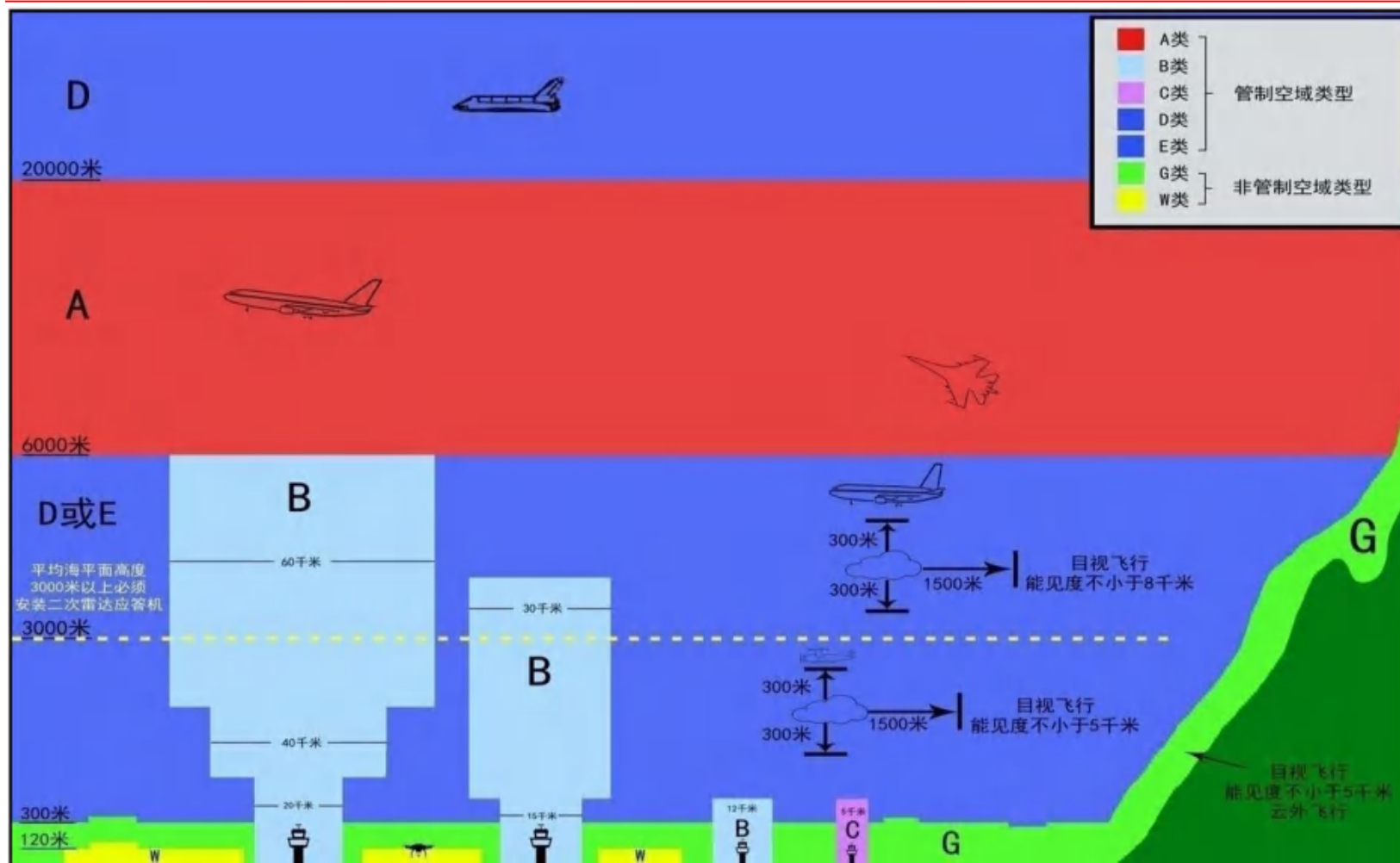
图2 国家空域基础分类示意图
